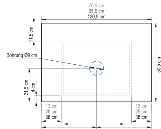
Bohrungen nur für den Waschtischabfluss
