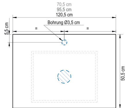
Bohrungen für Waschtischabfluss und Armatur
