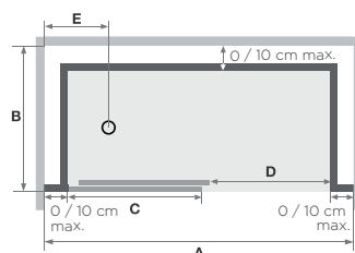
Montage en niche (inversion possible)
