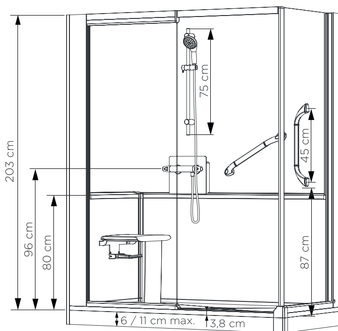
Kinemagic Royal : modèle en niche mi-haut - version avec thermostat - porte coulissante - verre avec partie centrale mate
