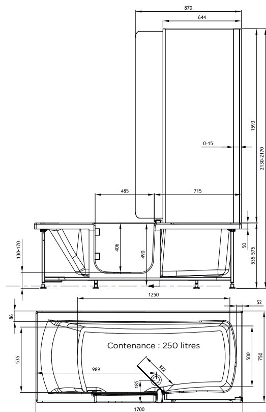
Version 170 x 80 cm, repose-tête à gauche
