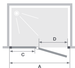
Tailles \geq 120 cm Installation au choix : à gauche ou à droite
