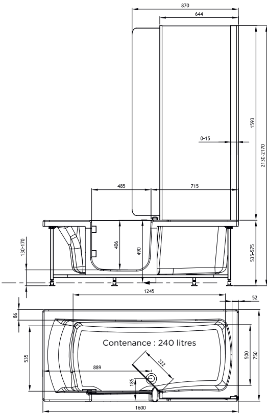
Version 160 x 80 cm, repose-tête à gauche
