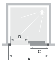
Élément fixe à droite, ouverture à gauche
