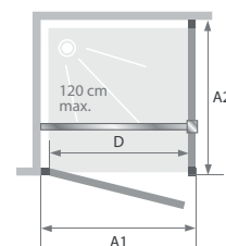
Tailles \leq 100 cm Installation au choix : à gauche ou à droite
