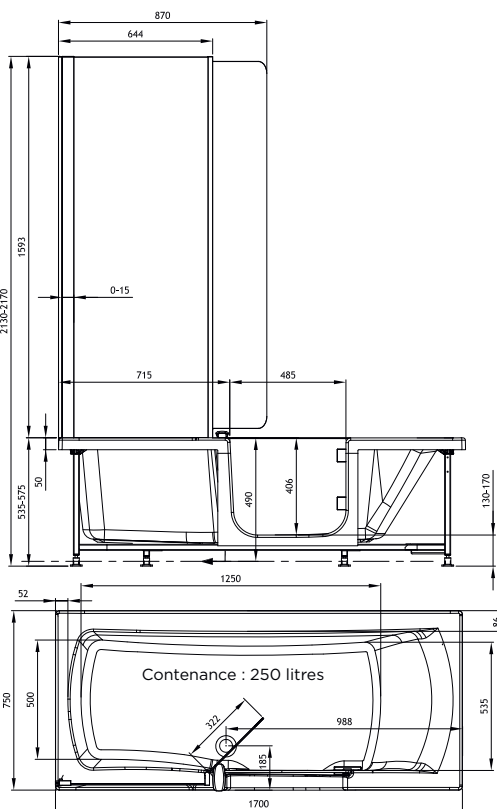
Version 170 x 80 cm, repose-tête à droite
