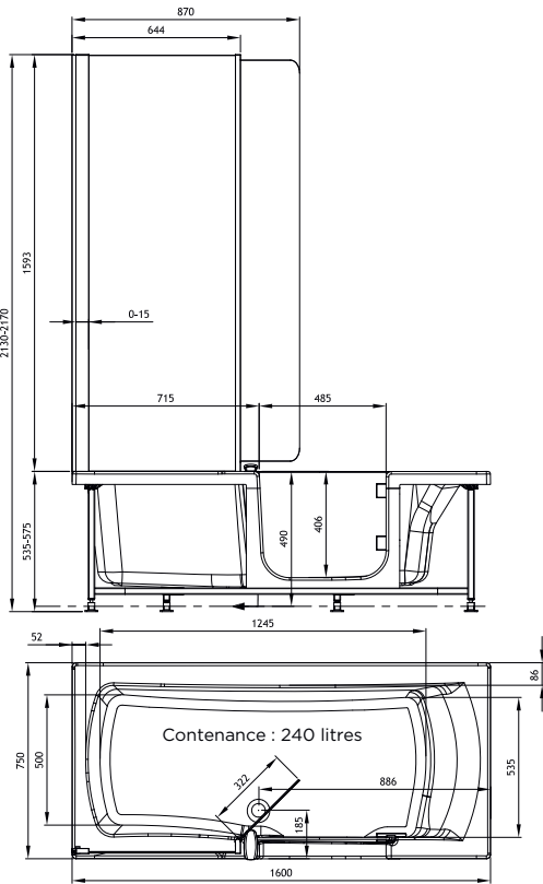
Version 160 x 80 cm, repose-tête à droite
