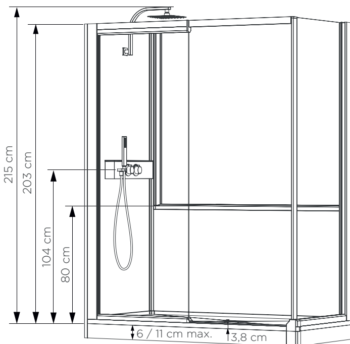
Kinemagic Design : modèle en niche mixte - version avec thermostat - porte coulissante - encastrement partiel
