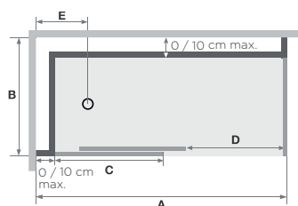
Montage d'angle (inversion possible)
