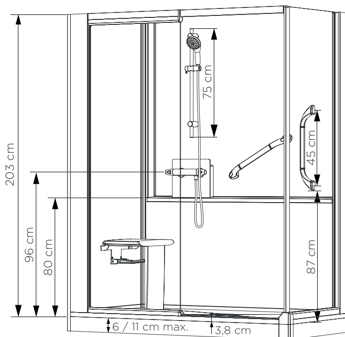
Kinemagic Royal : modèle en niche mixte - version avec mitigeur mécanique - espace douche ouvert
