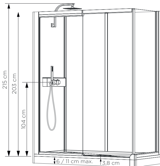
Kinemagic Design : modèle en niche haut - version avec mitigeur mécanique - porte coulissante - verre avec partie centrale mate - encastrement partiel
