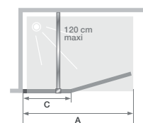
Tailles \geq 110 cm Installation au choix : à gauche ou à droite
