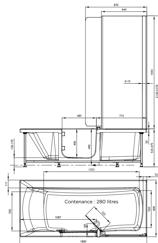
Version 180 x 80 cm, repose-tête à gauche
