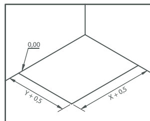
Vorbereitung montage
